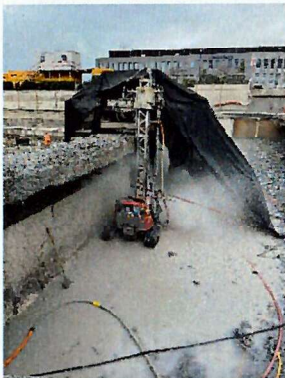
Roboter auf über 3.5m Arbeitshöhe
