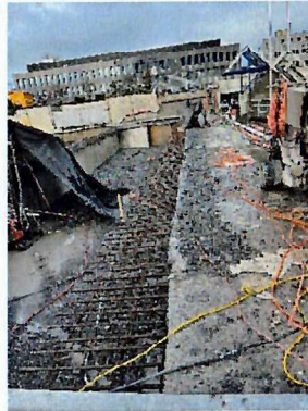
Komplette Deckenstärke T = 0.50m abgetragen.
